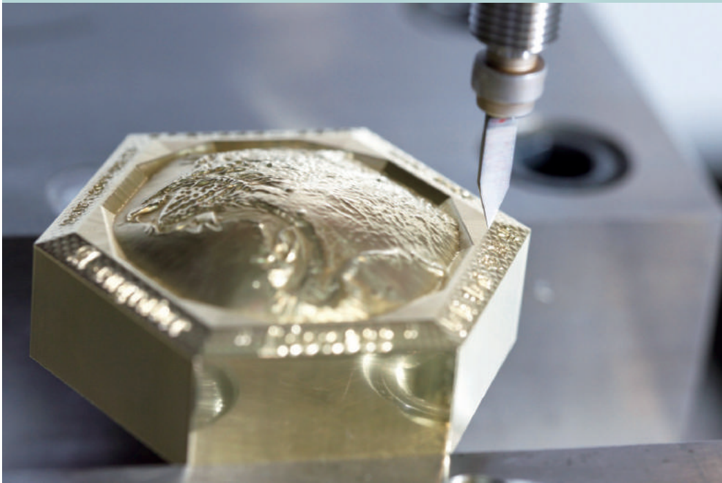
半月一枚刃を使った切削加工
